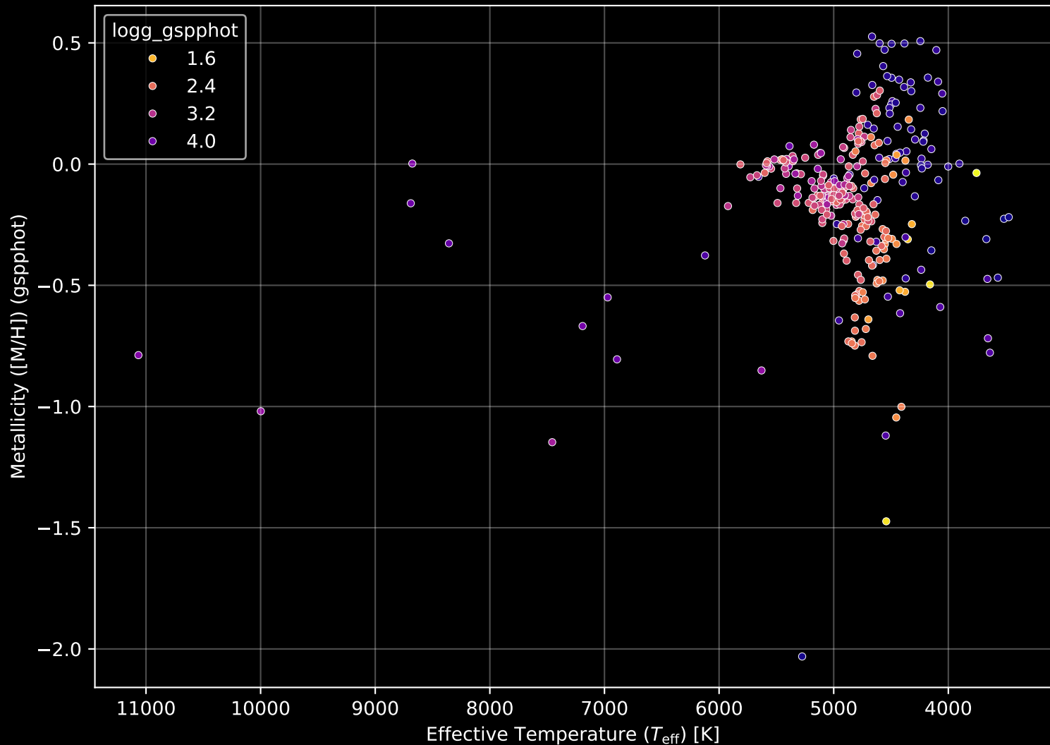
APOGEE DR17 Field: [140-24_btx] Stellar Population Parameters (n= 322)
